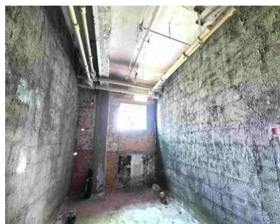
室内剔凿拆除施工
