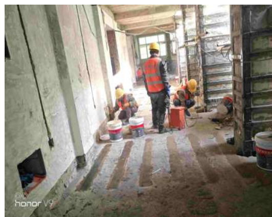
碳纤维加固施工
